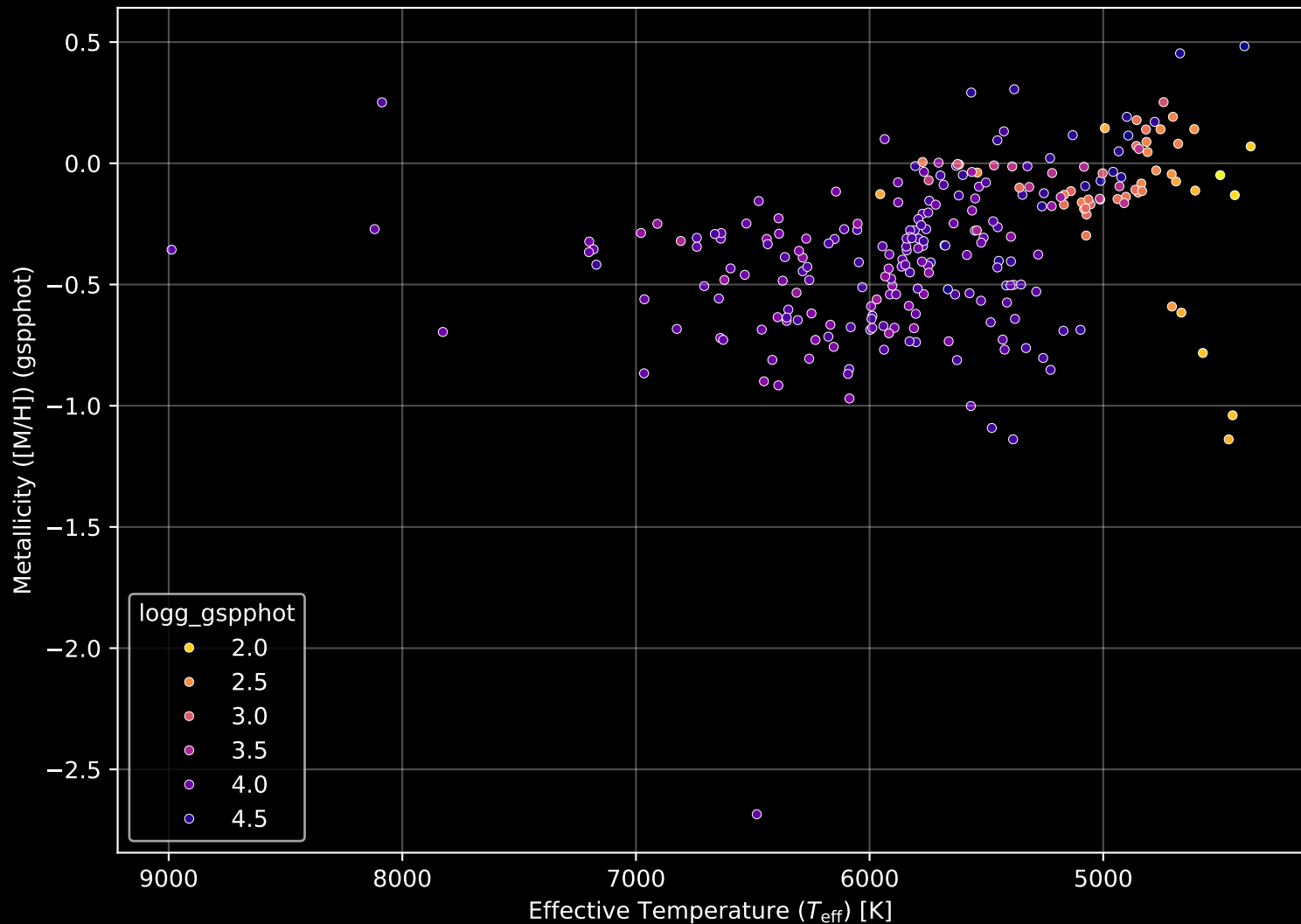
GALAH DR4 Field: [2422] Stellar Population Parameters (n= 254)
