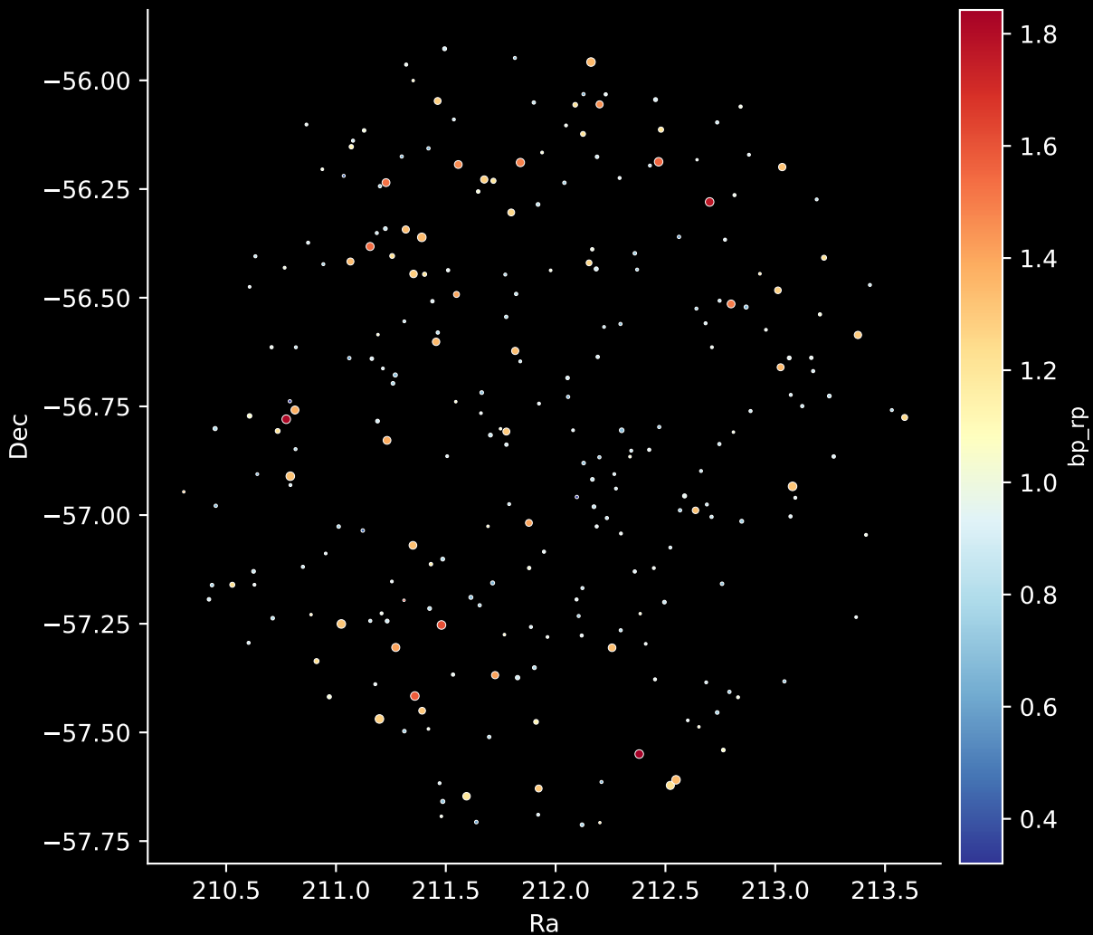
GALAH DR4 Field: [2422] Stars: 254
